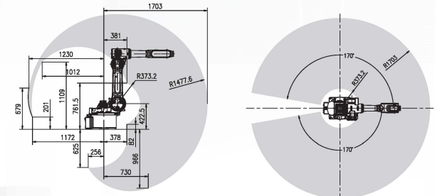
URB20A-1700 Motion range diagram
